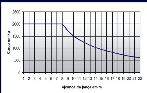
DIAGRAMA DE CARGAS
